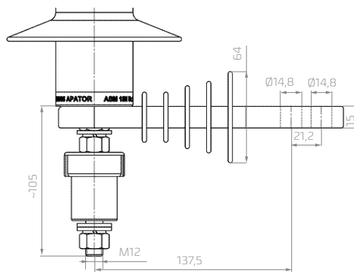
insulating bracket with disconnect Isolationsträger mit einem Trennschalter
