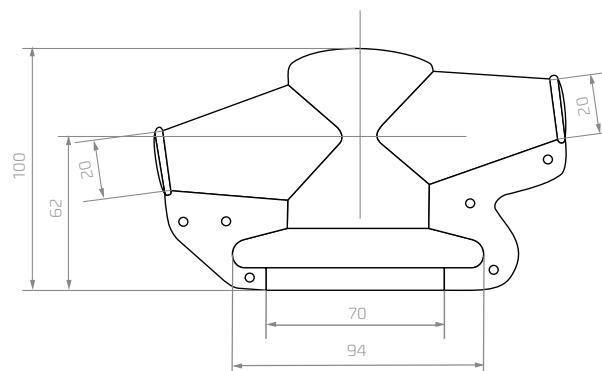
cover Gehäuse
