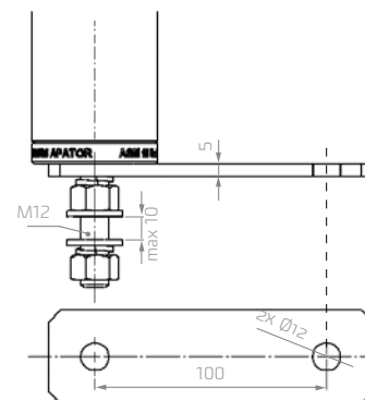
straight metal bracket einfacher Einbauträger
