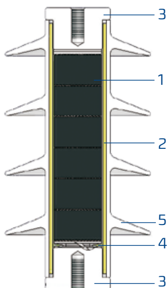
ASM 18N type surge arrester Überspannungsableiter Typ ASM 18N
