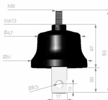
surge arrester version B Überspannungsableiter Ausführung B
