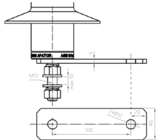
straight metal bracket einfacher Einbauträger
