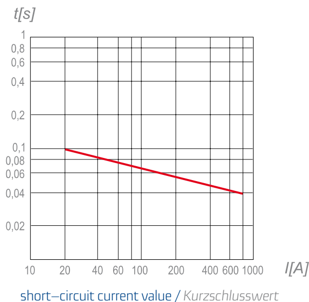
Diagram no. 1. Time versus current characteristics of a disconnecter Diagramm 1. Zeit-Strom-Kennlinie des Trennschalters
