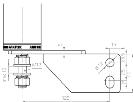
angle metal bracket Einbauwinkel
