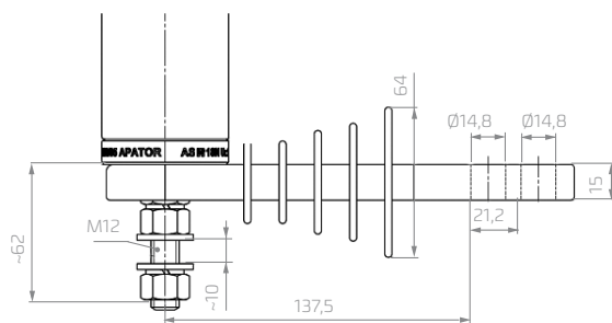
insulating bracket Isolationsträger
