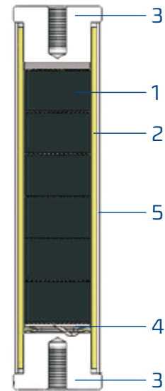
ASW 18 type surge arrester Überspannungsableiter Typ ASW 18
