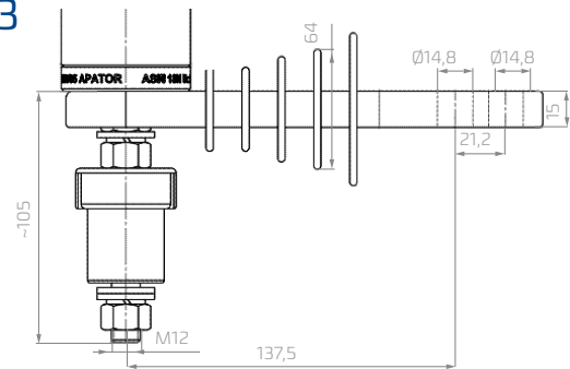
insulating bracket with disconnector Isolationsträger mit einem Trennschalter
