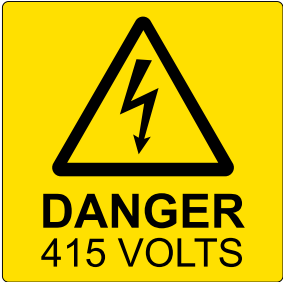
SL5050D415
